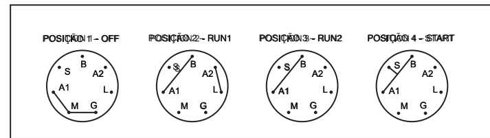
POSICÕES DO COMUTADOR DE CHAVES
